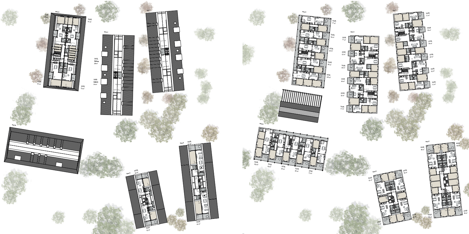
Grundrisse Dachgeschoss
