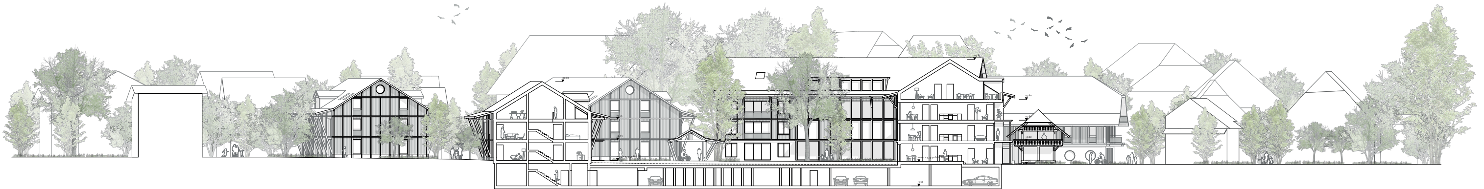
Schnitt-Ansicht Ost-West (von Norden)
