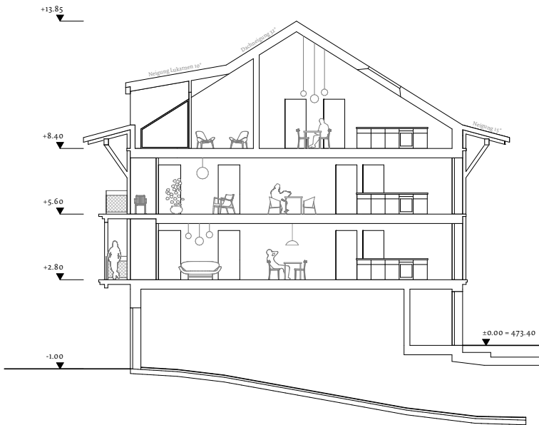
Querschnitt
