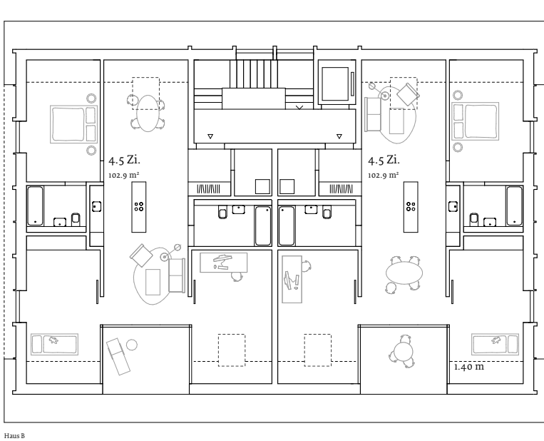
Grundriss Dachgeschoss
