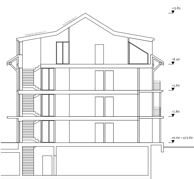
Querschnitt
