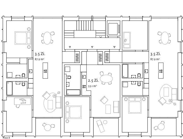
Grundriss 2. Obergeschoss
