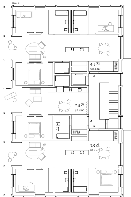
Grundriss 1. Obergeschoss
