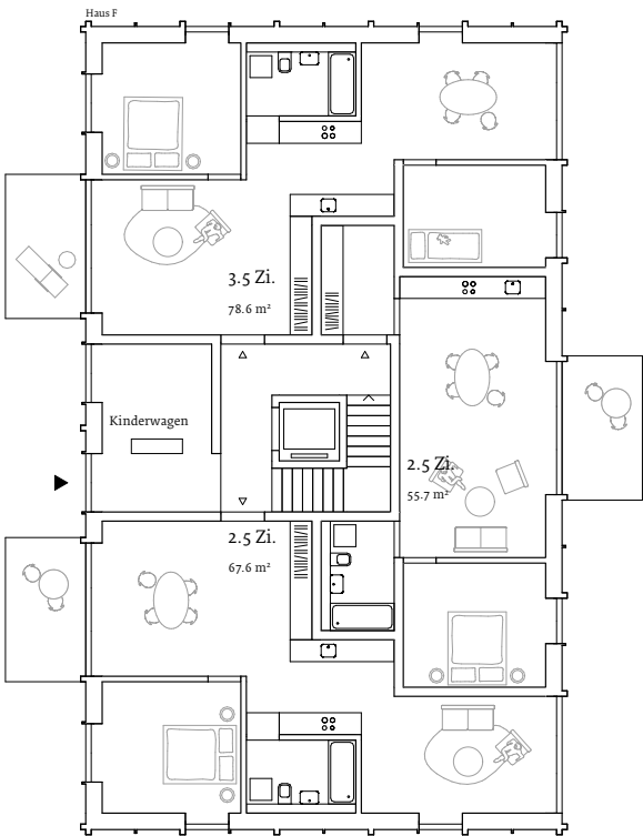
Grundriss Erdgeschoss
