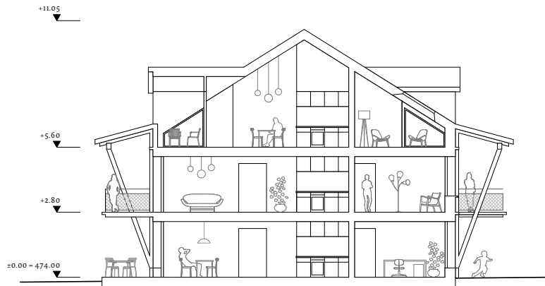
Querschnitt
