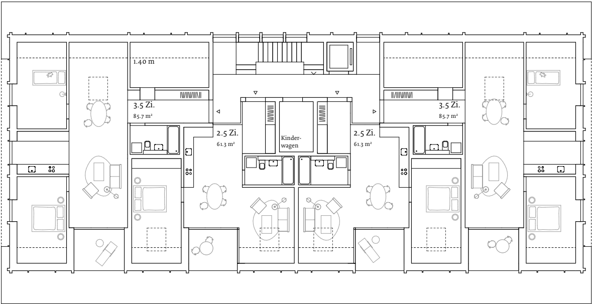
Grundriss Dachgeschoss
