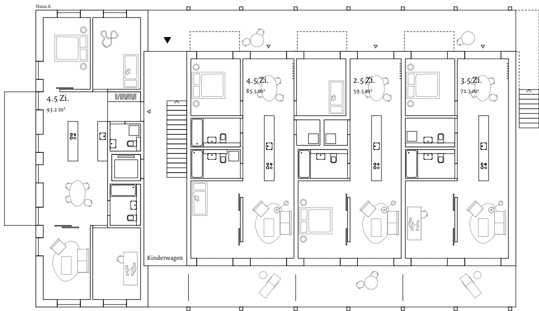
Grundriss Erdgeschoss
