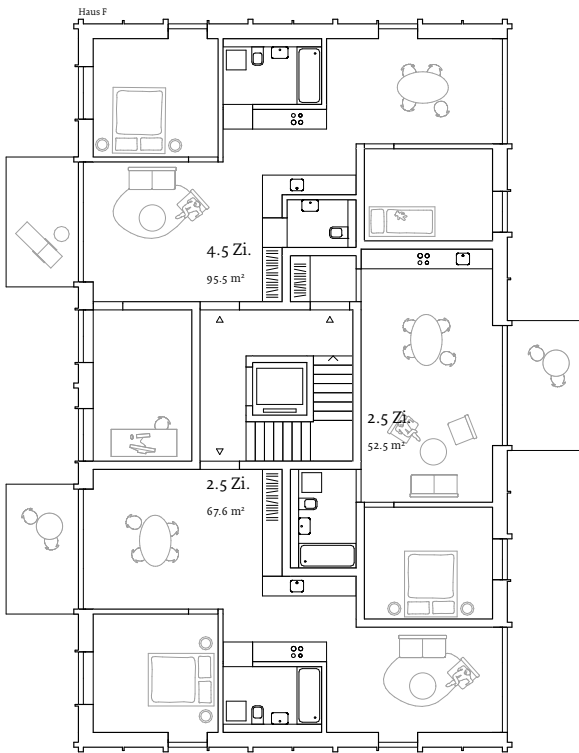
Grundriss 1. Obergeschoss
