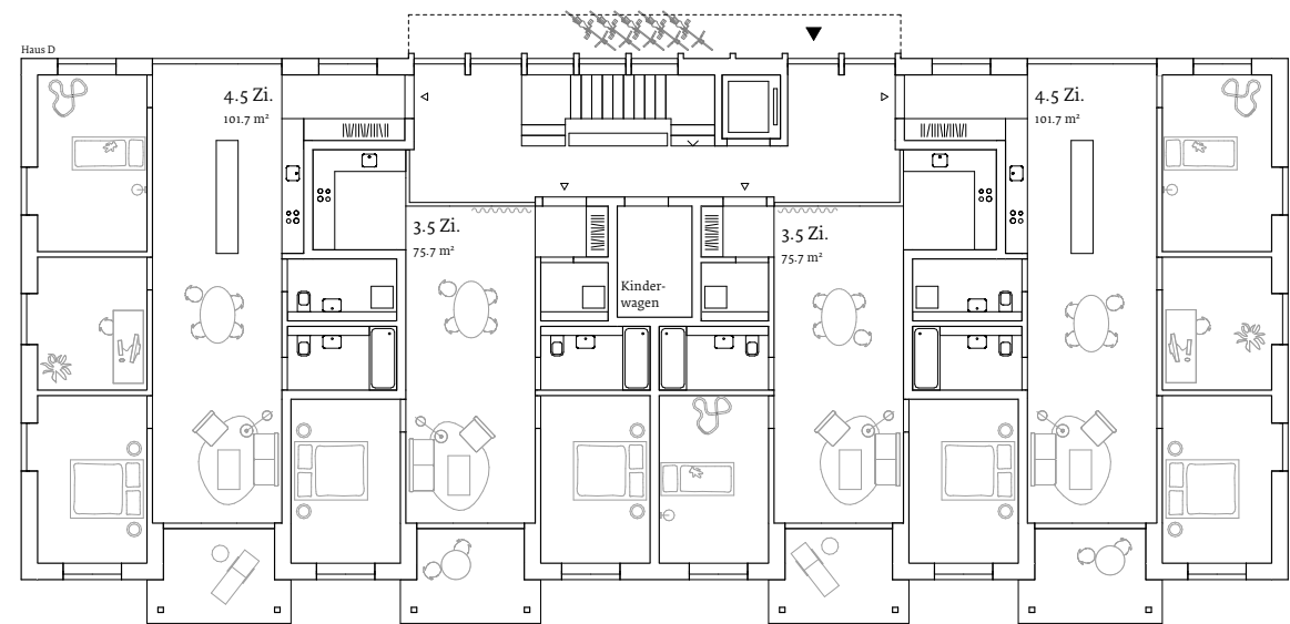
Grundriss Erdgeschoss
