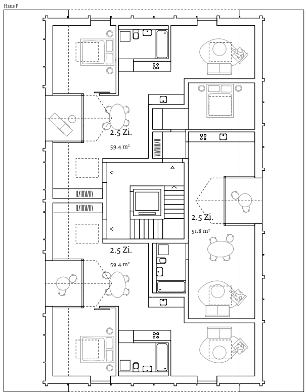
Grundriss Dachgeschoss
