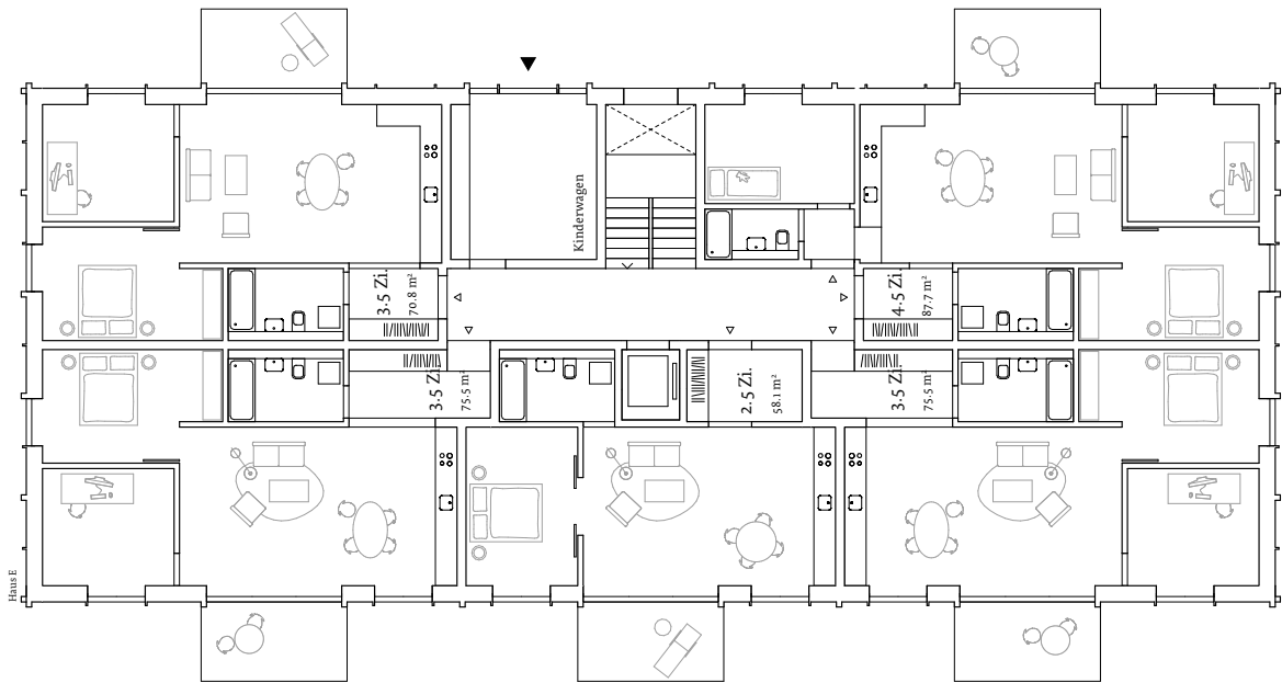
Grundriss Erdgeschoss
