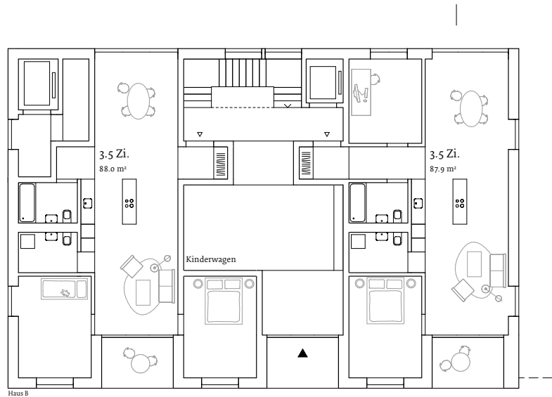
Grundriss Erdgeschoss
