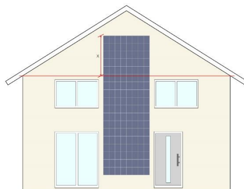
Abb. 27 Die Anlage ragt in die Giebelfläche hinein und deckt diese nicht vollständig ab.
