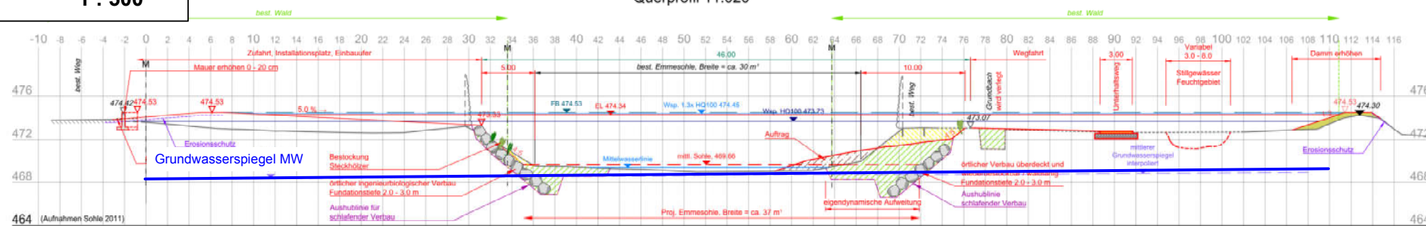
Querprofil 11.020
